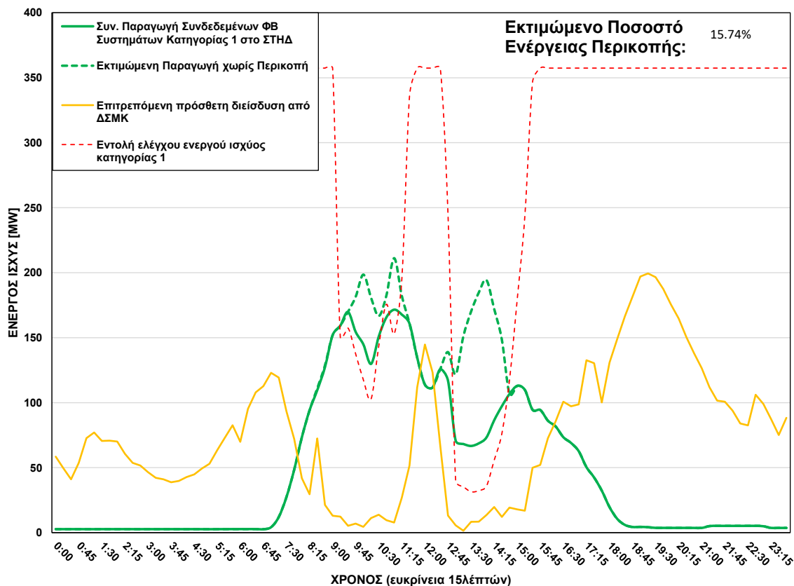
ΦΒ Παραγωγή στο ΣΤΗΔ στις 30/09/2026 (ώρα περικοπής: 09:00 - 14:30)
