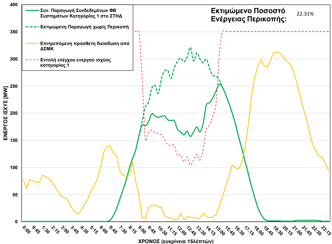
ΦΒ Παραγωγή στο ΣΤΗΔ στις 15/09/2026 (ώρα περικοπής: 09:15 - 15:15)
