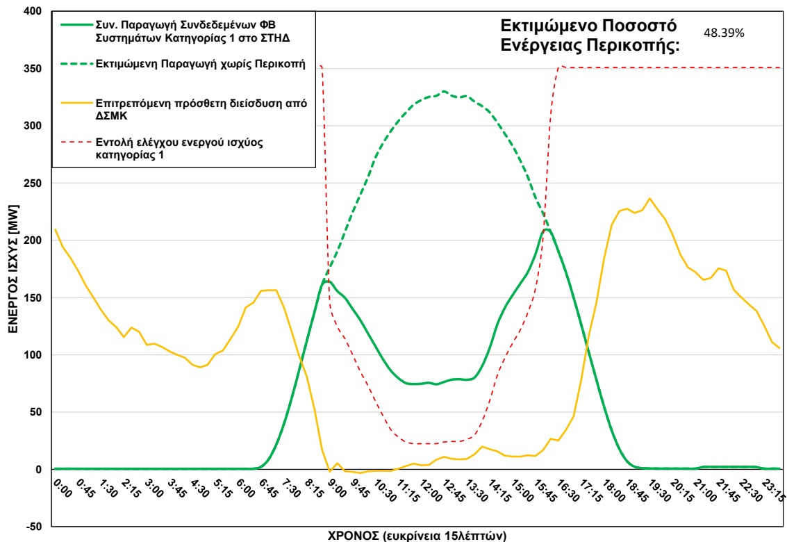
ΦΒ Παραγωγή στο ΣΤΗΔ στις 11/09/2026 (ώρα περικοπής: 09:00 - 16:00)
