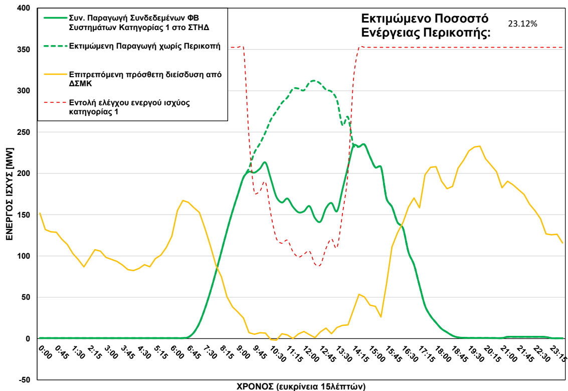
ΦΒ Παραγωγή στο ΣΤΗΔ στις 17/09/2026 (ώρα περικοπής: 09:30 - 14:00)
