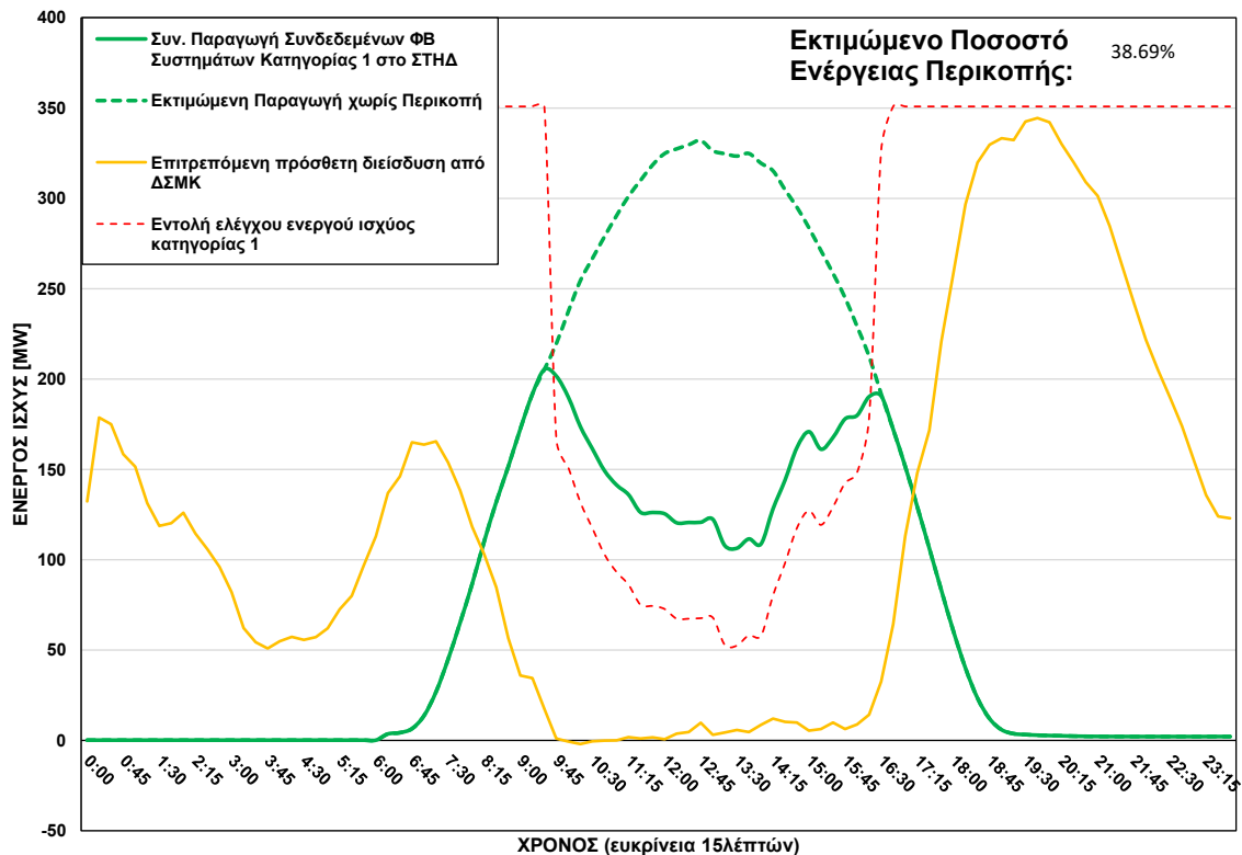
ΦΒ Παραγωγή στο ΣΤΗΔ στις 08/09/2026 (ώρα περικοπής: 09:30 - 16:15)
