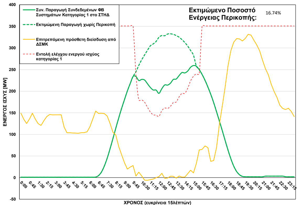
ΦΒ Παραγωγή στο ΣΤΗΔ στις 02/09/2026 (ώρα περικοπής: 10:00 - 15:00)
