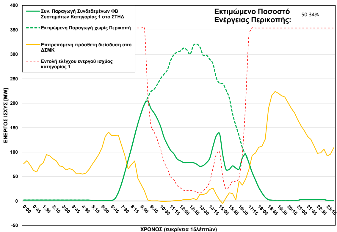
ΦΒ Παραγωγή στο ΣΤΗΔ στις 23/09/2026 (ώρα περικοπής: 09:30 - 16:45)
