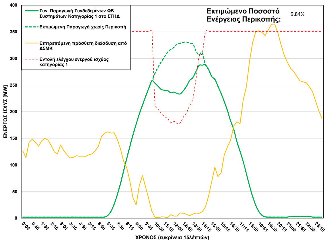
ΦΒ Παραγωγή στο ΣΤΗΔ στις 03/09/2026 (ώρα περικοπής: 10:15 - 14:15)
