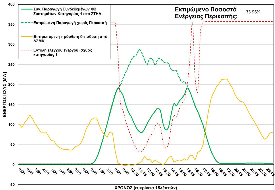
ΦΒ Παραγωγή στο ΣΤΗΔ στις 24/09/2026 (ώρα περικοπής: 09:15 - 15:45)
