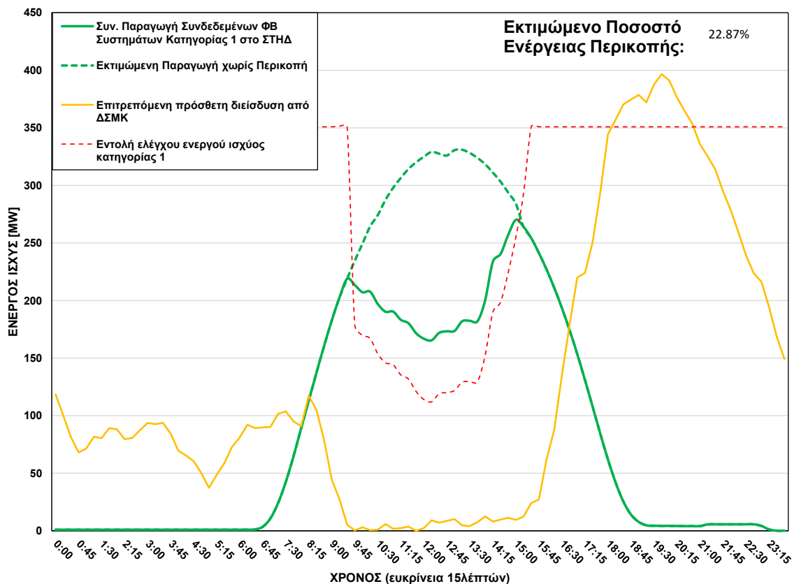
ΦΒ Παραγωγή στο ΣΤΗΔ στις 07/09/2026 (ώρα περικοπής: 09:30 - 15:00)
