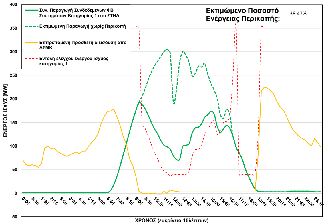
ΦΒ Παραγωγή στο ΣΤΗΔ στις 21/09/2026 (ώρα περικοπής: 09:15 - 16:30)
