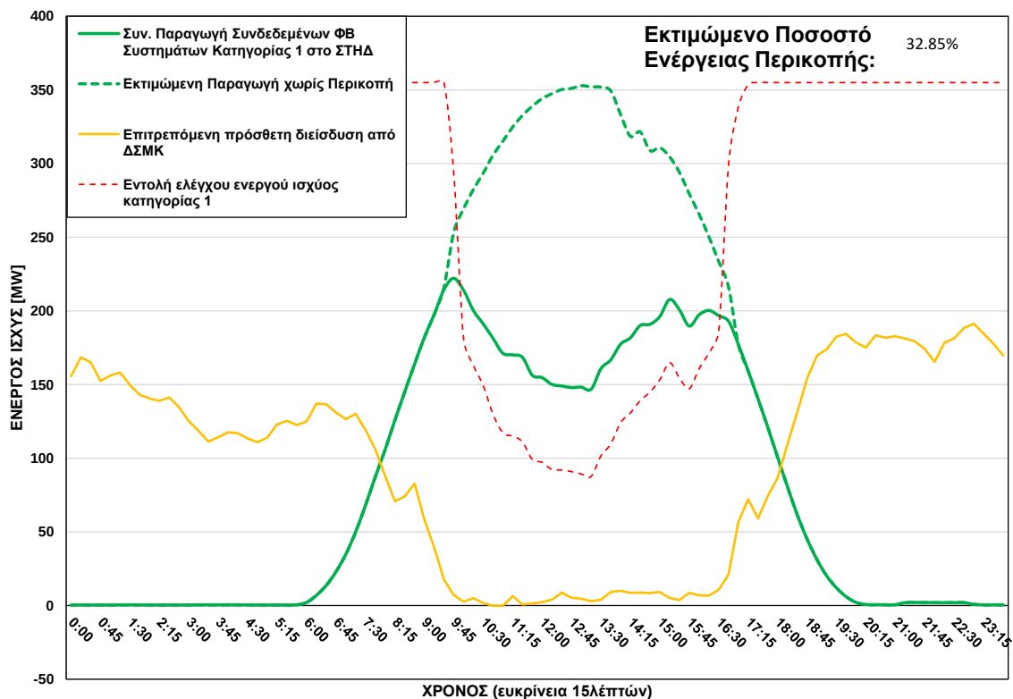
ΦΒ Παραγωγή στο ΣΤΗΔ στις 03/07/2026 (ώρα περικοπής: 09:45 - 16:45)
