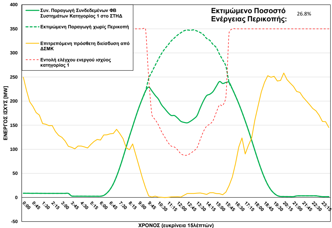
ΦΒ Παραγωγή στο ΣΤΗΔ στις 31/07/2026 (ώρα περικοπής: 09:45 - 15:45)
