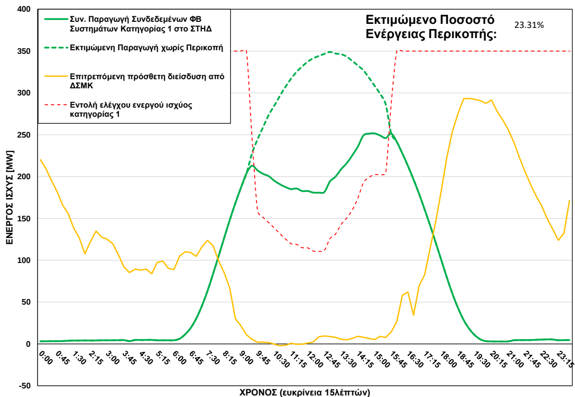
ΦΒ Παραγωγή στο ΣΤΗΔ στις 29/07/2026 (ώρα περικοπής: 09:30 - 15:30)
