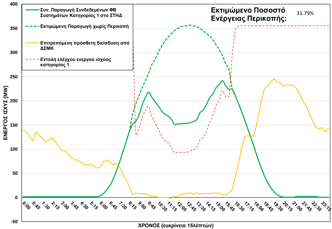
ΦΒ Παραγωγή στο ΣΤΗΔ στις 02/07/2026 (ώρα περικοπής: 08:30 - 16:00)
