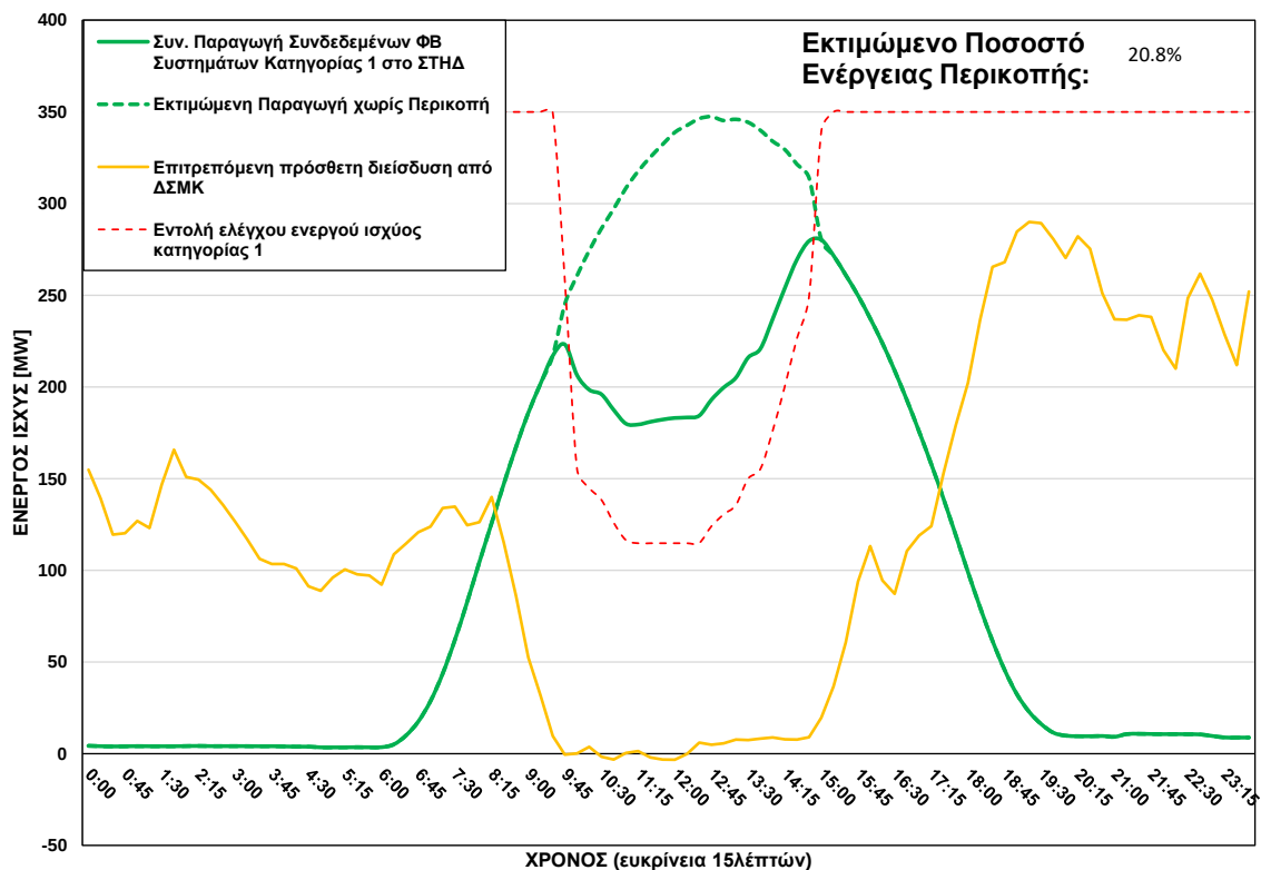
ΦΒ Παραγωγή στο ΣΤΗΔ στις 30/07/2026 (ώρα περικοπής: 09:45 - 14:45)
