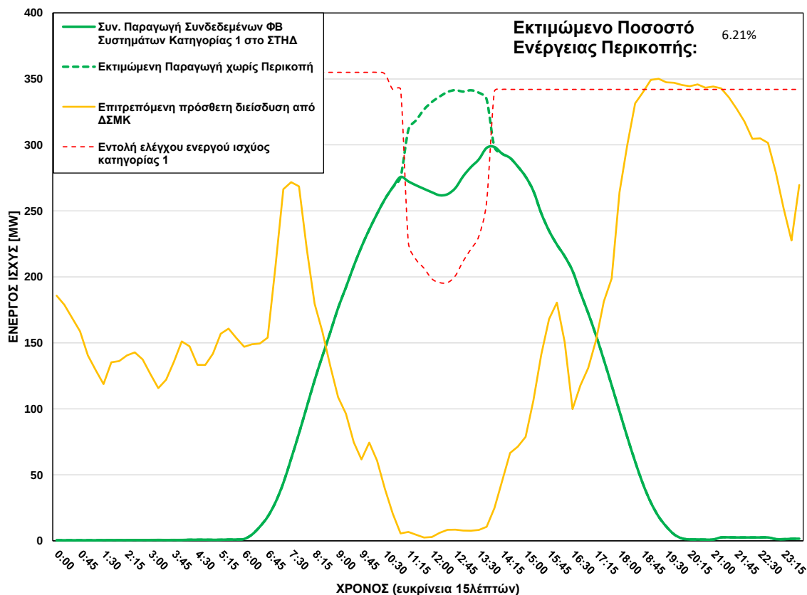
ΦΒ Παραγωγή στο ΣΤΗΔ στις 21/07/2026 (ώρα περικοπής: 11:15 - 13:45)
