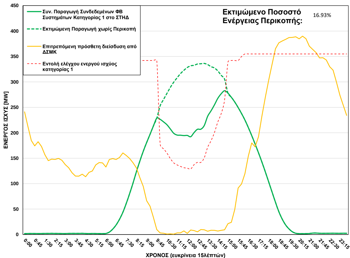
ΦΒ Παραγωγή στο ΣΤΗΔ στις 22/07/2026 (ώρα περικοπής: 10:00 - 14:45)
