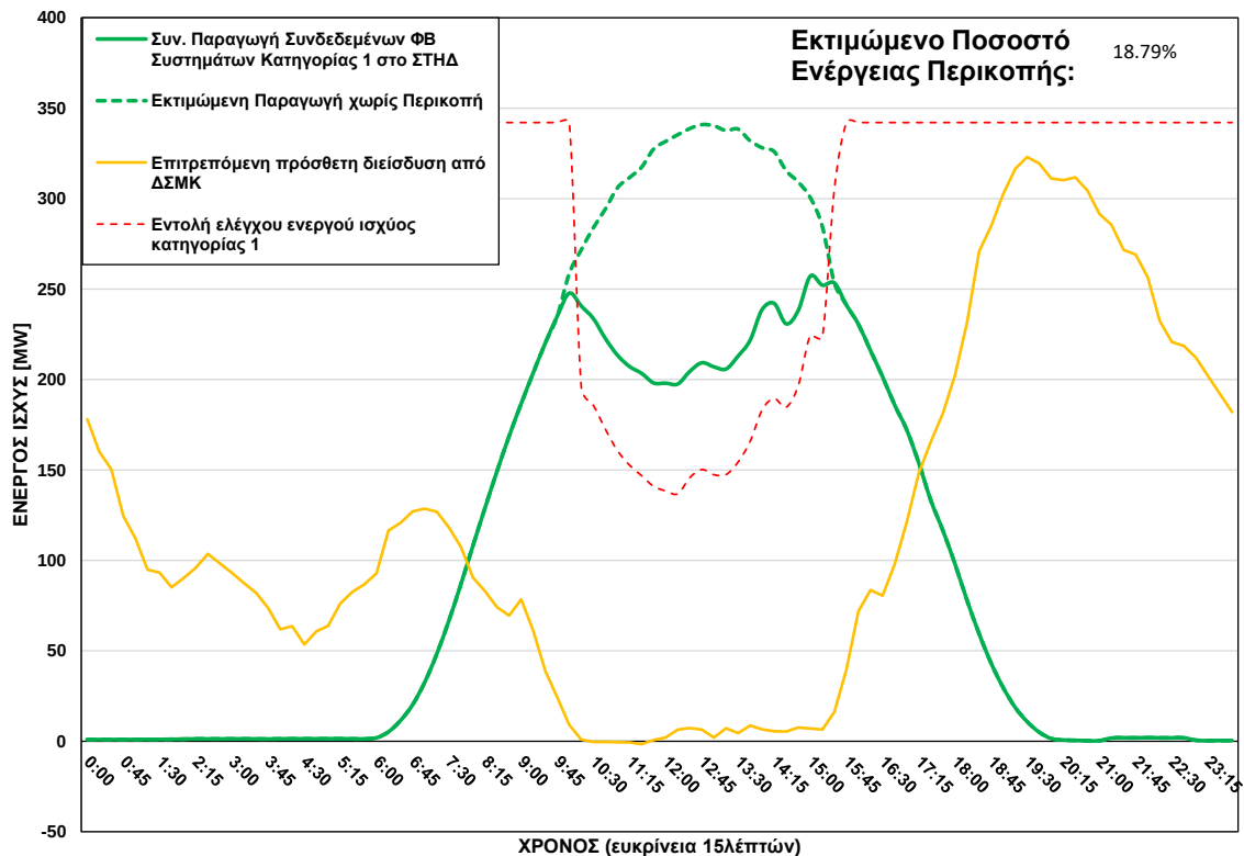
ΦΒ Παραγωγή στο ΣΤΗΔ στις 17/07/2026 (ώρα περικοπής: 10:00 - 15:15)
