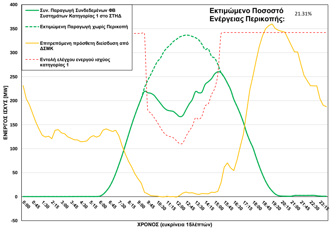
ΦΒ Παραγωγή στο ΣΤΗΔ στις 16/07/2026 (ώρα περικοπής: 09:30 - 15:15)
