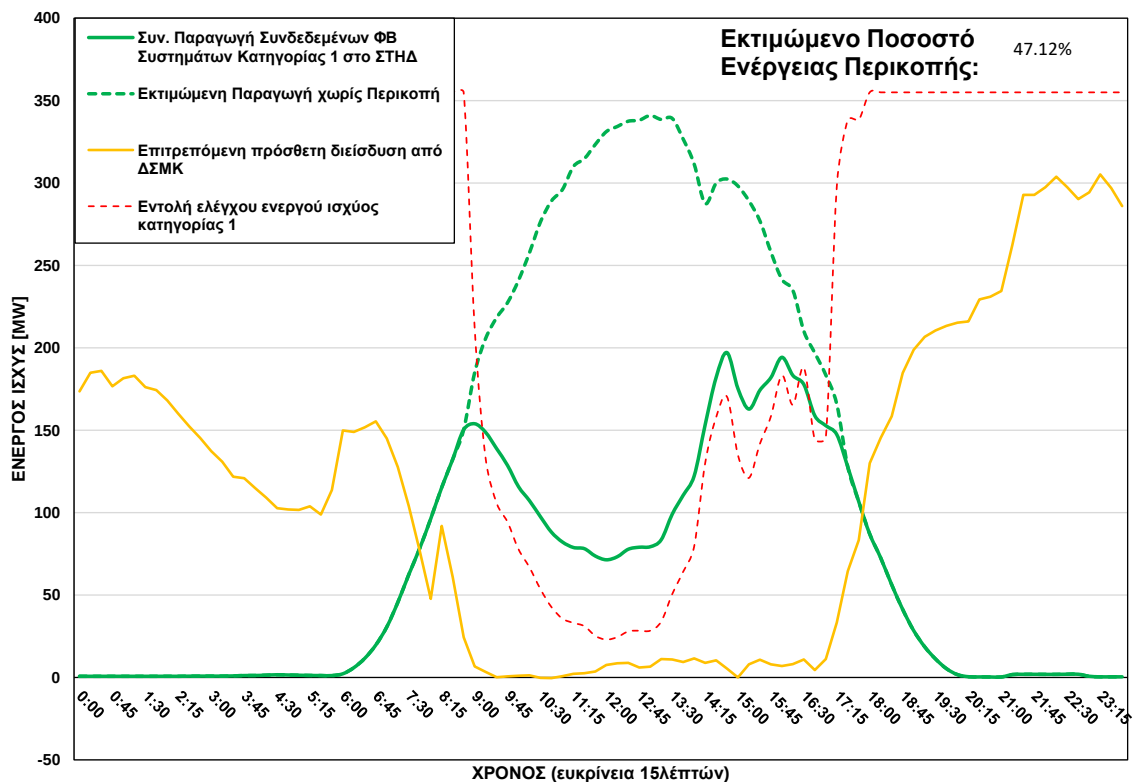
ΦΒ Παραγωγή στο ΣΤΗΔ στις 05/07/2026 (ώρα περικοπής: 09:00 - 17:15)
