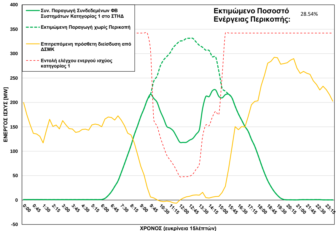
ΦΒ Παραγωγή στο ΣΤΗΔ στις 24/07/2026 (ώρα περικοπής: 10:00 - 15:30)
