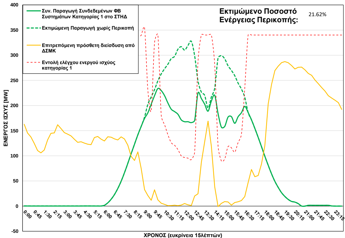
ΦΒ Παραγωγή στο ΣΤΗΔ στις 07/07/2026 (ώρα περικοπής: 09:15 - 16:30)
