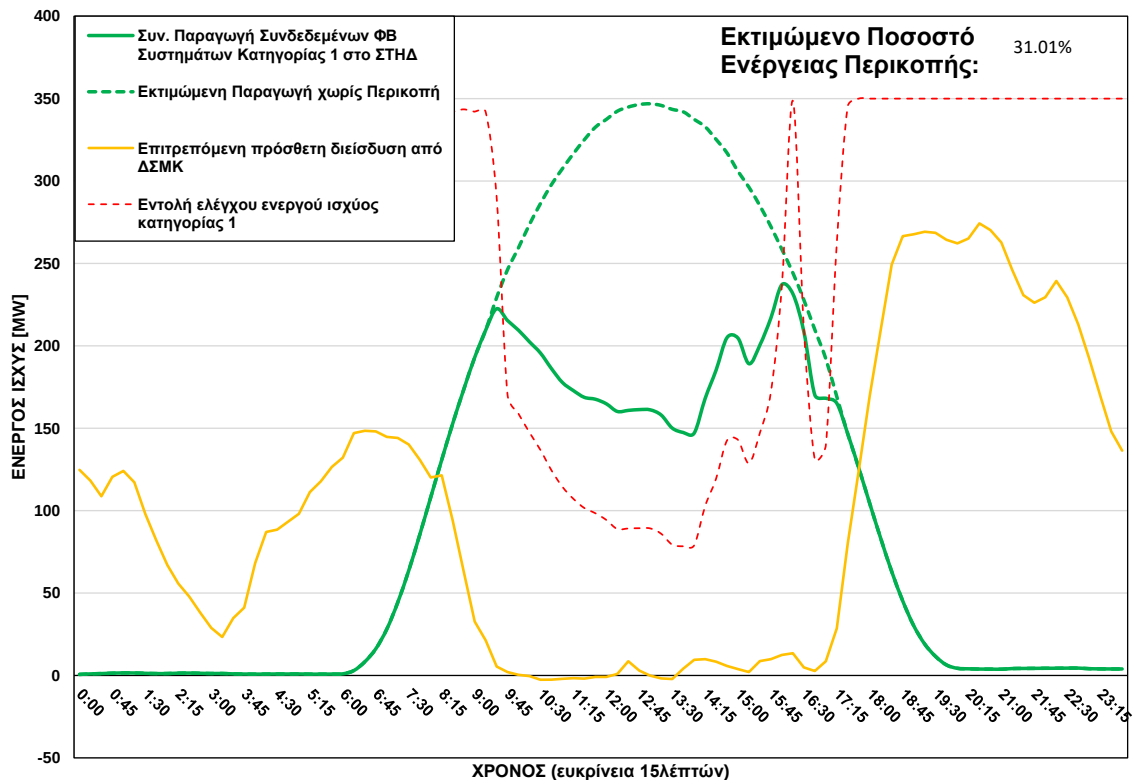
ΦΒ Παραγωγή στο ΣΤΗΔ στις 27/07/2026 (ώρα περικοπής: 09:30 - 17:15)
