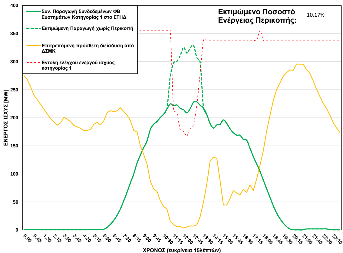
ΦΒ Παραγωγή στο ΣΤΗΔ στις 06/07/2026 (ώρα περικοπής: 11:00 - 13:15)
