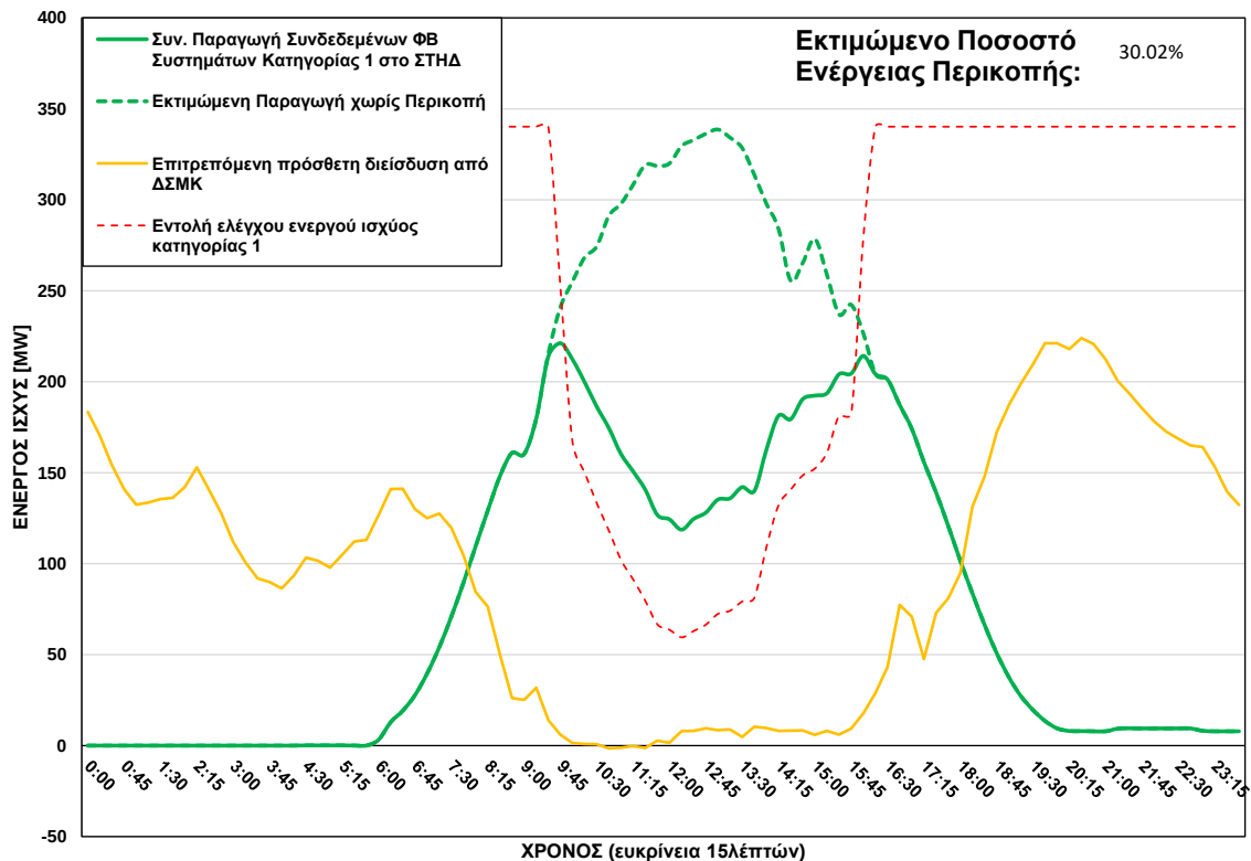
ΦΒ Παραγωγή στο ΣΤΗΔ στις 08/07/2026 (ώρα περικοπής: 09:45 - 16:00)
