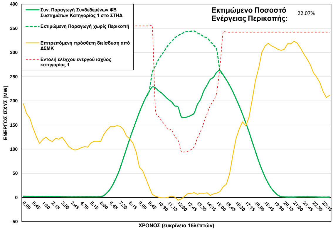
ΦΒ Παραγωγή στο ΣΤΗΔ στις 23/07/2026 (ώρα περικοπής: 10:00 - 15:00)
