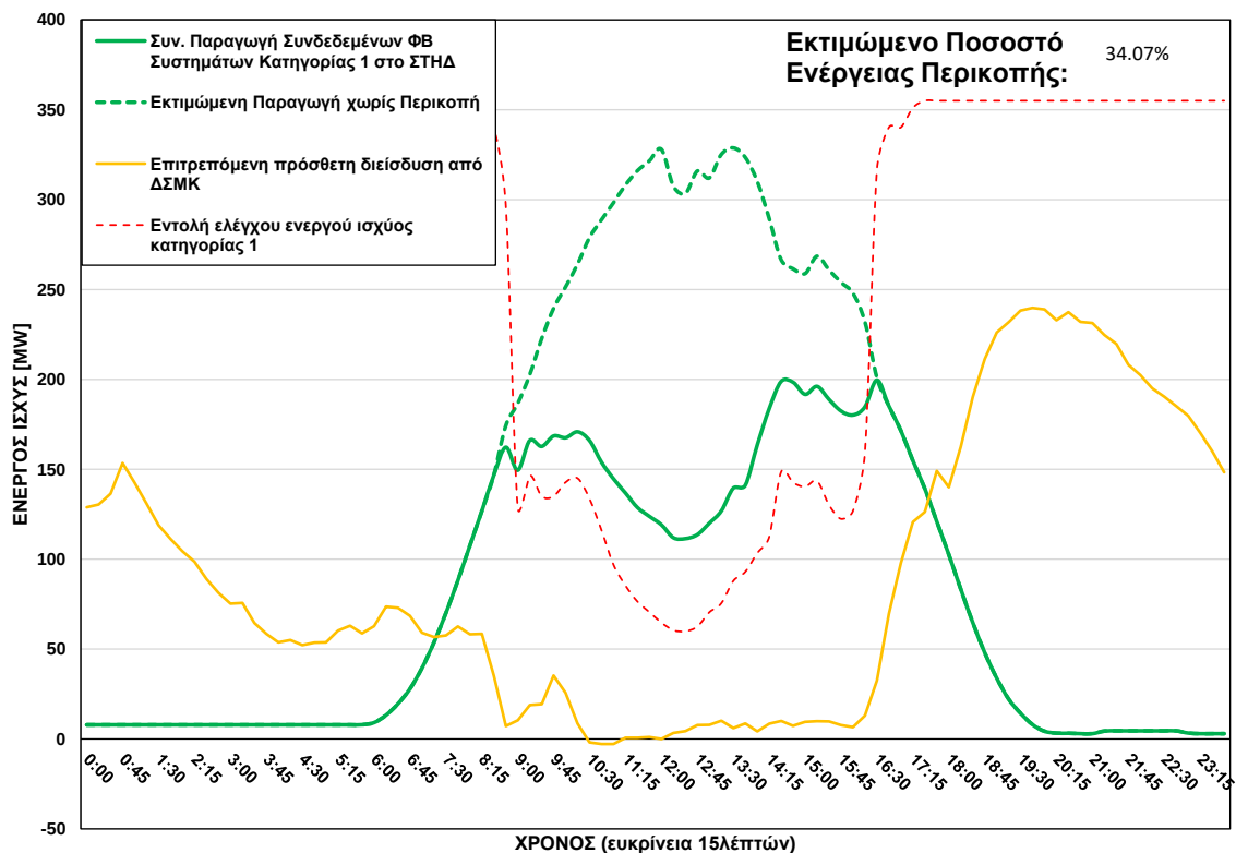
ΦΒ Παραγωγή στο ΣΤΗΔ στις 09/07/2026 (ώρα περικοπής: 08:45 - 16:15)
