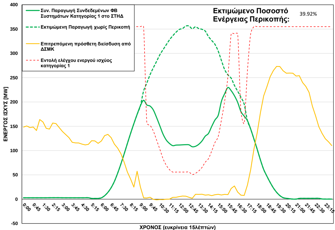
ΦΒ Παραγωγή στο ΣΤΗΔ στις 10/07/2026 (ώρα περικοπής: 09:15 - 17:00)
